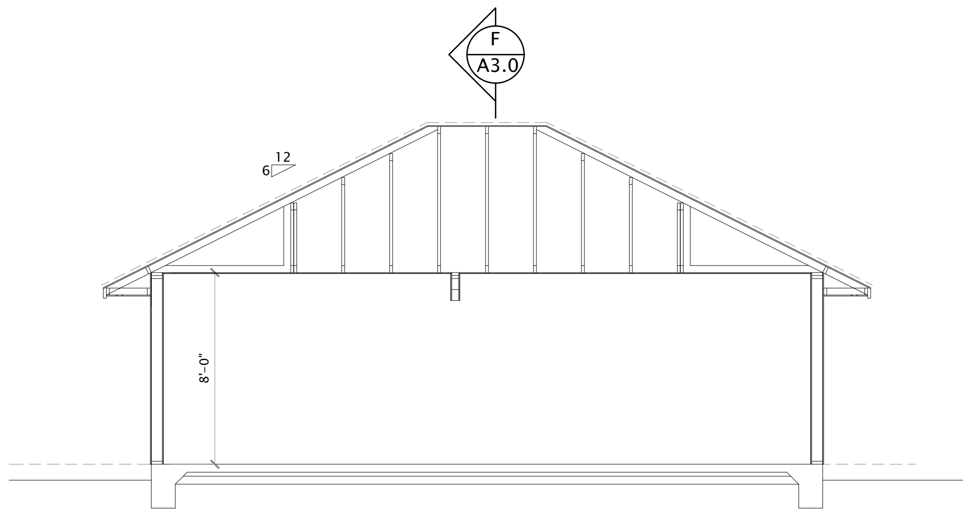
E SECTION SCALE: 1/4" = 1'-0"
