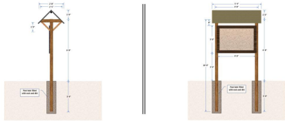
Kiosk Design
